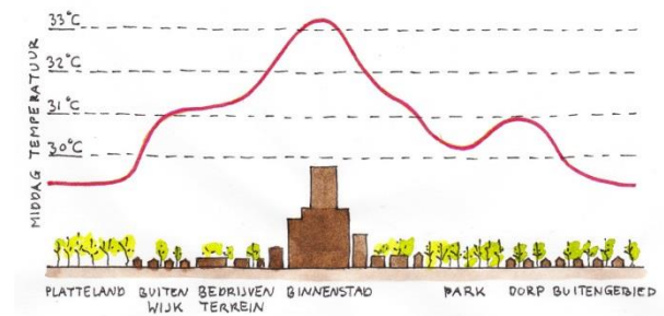
hitte-eiland-effect
